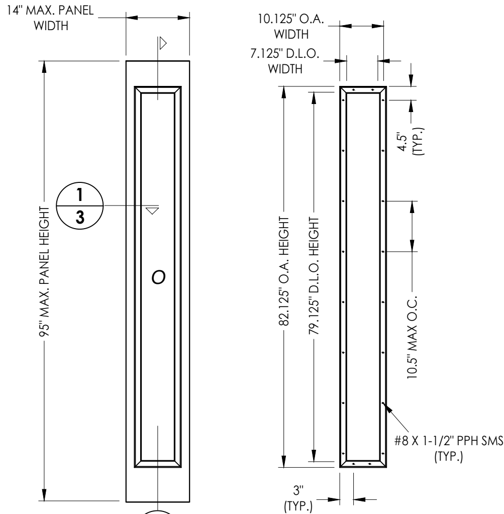
ODL LITE FRAME
